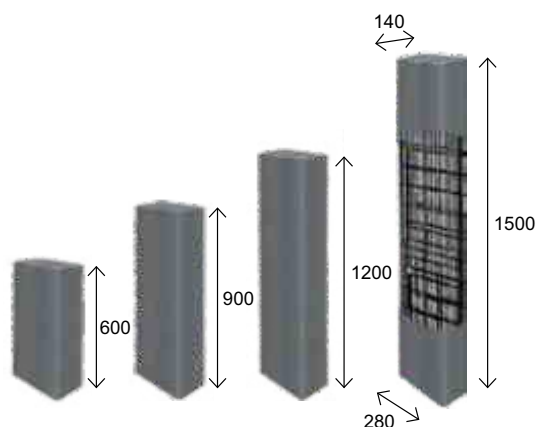
Palisáda 1500 mm armovaná
