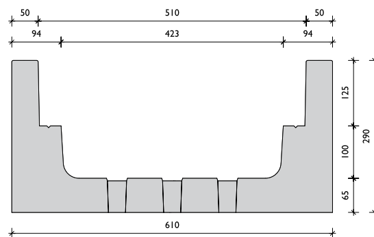
BG Káblový žľab KKv3 s vloženým krytom a falcom 125 mm
