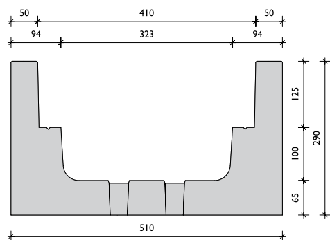
BG – Káblový žľab KKv2 s vloženým krytom a falcom 125 mm
