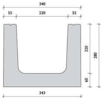
BG KV betónový kryt Gr. 3
