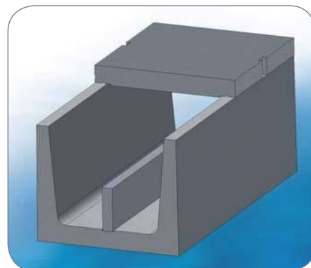
Deliacej stienky v Káblovom žľabe WL 413/335 slúžia na oddelenie rôznych káblov
