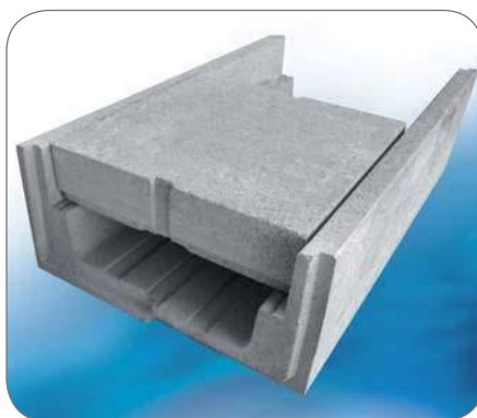
Kryt káblového žľabu zabezpečuje svojou výškou 125 mm zvýšenú protipožiarnu bezpečnosť.
