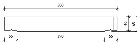
Krycia doska Gr. 3
