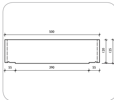
Priečny rez krytom BG Káblového žľabu KKv3 s falcom 125 mm
