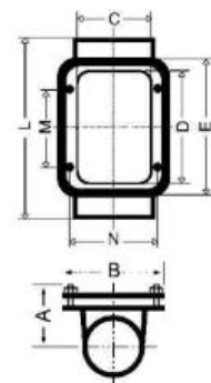
Čistící kus
