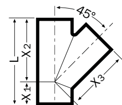
Odbočka 45°
