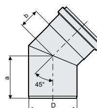
Tvar kolena D = 200.
