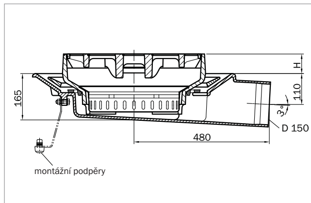
Vpust s přímým bočním odtokem:
