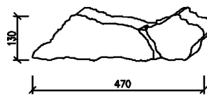
Krajový prvok B
