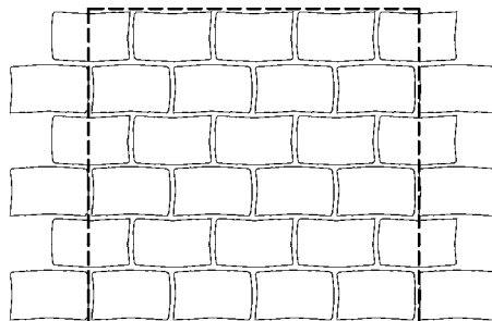
ALT-p04 9,18 ks/m 2 – normál 18,37 ks/m 2 – jeden a pol
