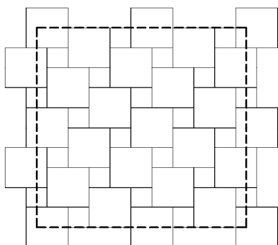
KLA-p13 11,11 ks/m 2 – 20/20 22,22 ks/m 2 – 20/10 (normál) 11,11 ks/m 2 – 10/10 (polovička)
