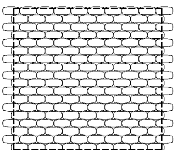
ROM-p03 152,56 ks/m 2 – polovička
