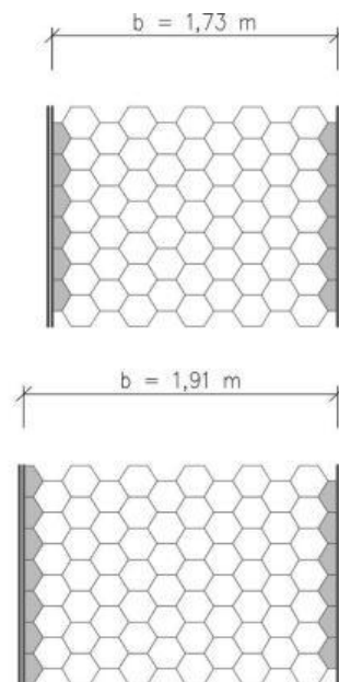
SEK-ch03 Príklady riešenia chodníkov na rôzne uhly zalomenia. Okraje sa riešia buď pomocou tvaroviek polovička, alebo rozpolením tvaroviek normál.
