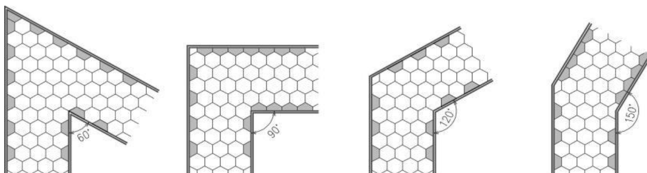
SEK-ch03 Príklady riešenia chodníkov na rôzne uhly zalomenia. Okraje sa riešia buď pomocou tvaroviek polovička, alebo rozpolením tvaroviek normál.
