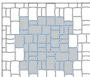
Vzor pokládky ALT-p13
