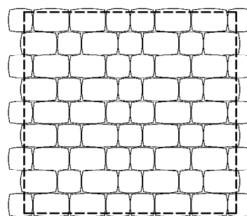
ROM-p06 30,30 ks/m 2 – normál 30,30 ks/m 2 – jeden a pol
