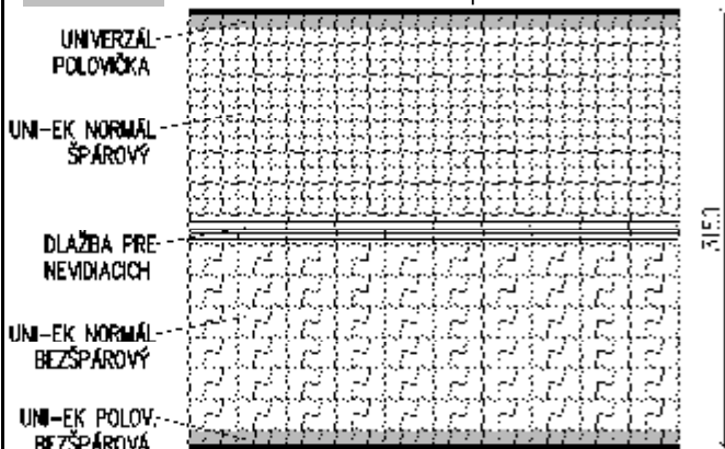
UNI-EK Príklad riešenia nástupišt'a
