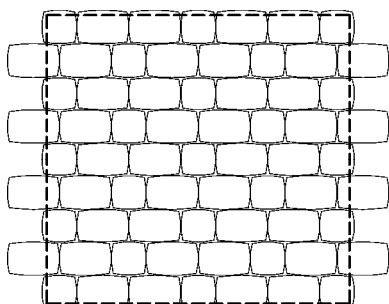
ROM-p07 18,94 ks/m 2 – normál 37,89 ks/m 2 – jeden a pol
