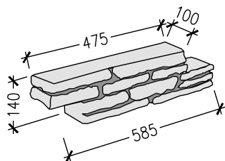
Z - blok 58,5 x 10 x 14 cm
